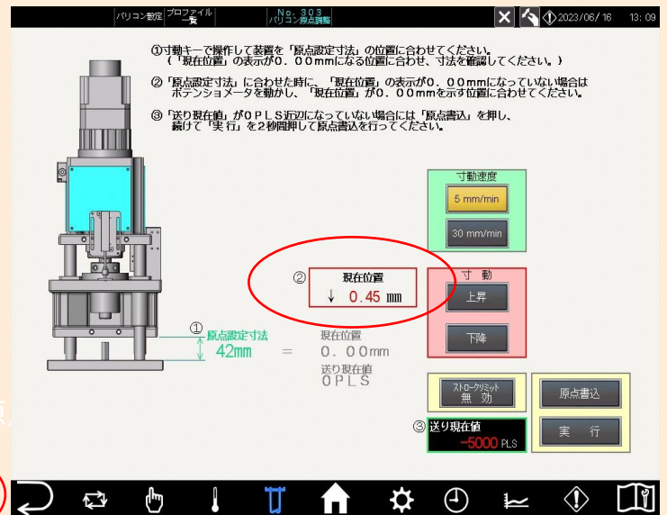
図②.No.303パリコン原点設定(Ver.6以降)
