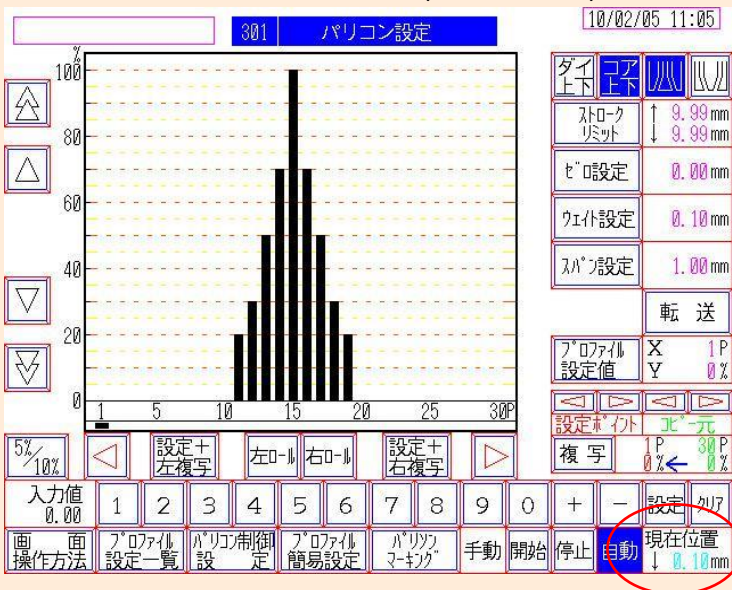
図①.No.301パリコン設定(Ver.4、Ver.5)
