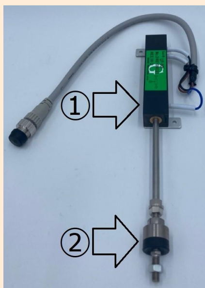
写真2： ①ポテンショメータ ②フローティングジョイント
